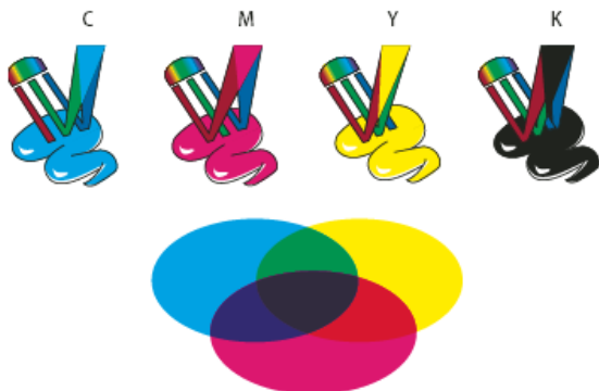
Субтрактивні кольори (СМΥК)
