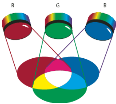
Аддитивні кольори (RGB)
