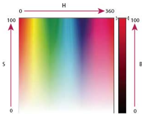
Колірна модель HSB
